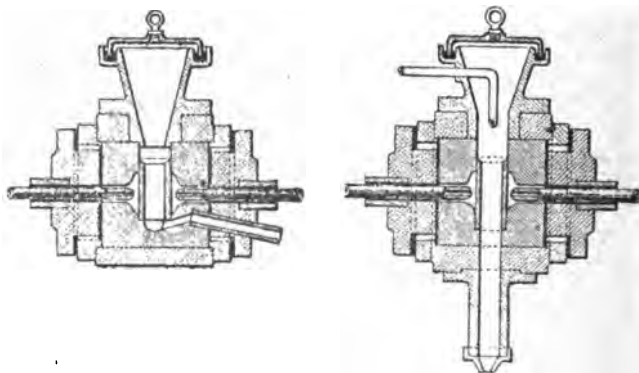
Fig. 156 et 157. — Fours Girard et Street.
